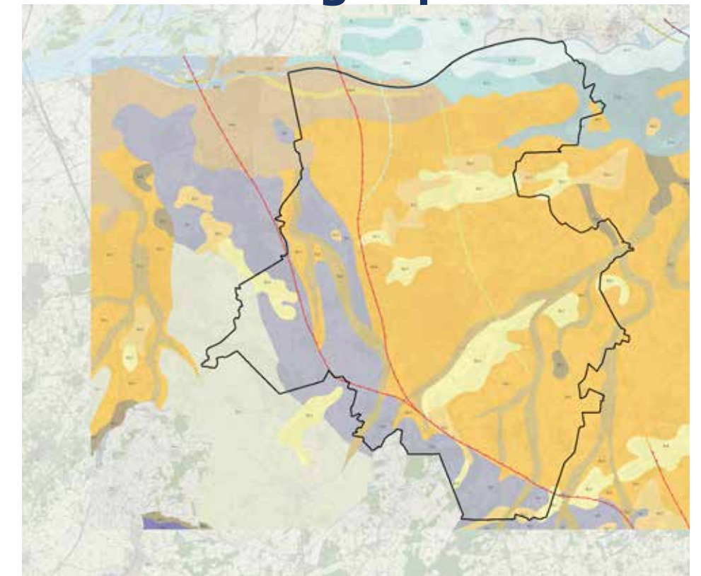
Geologie en breuken
