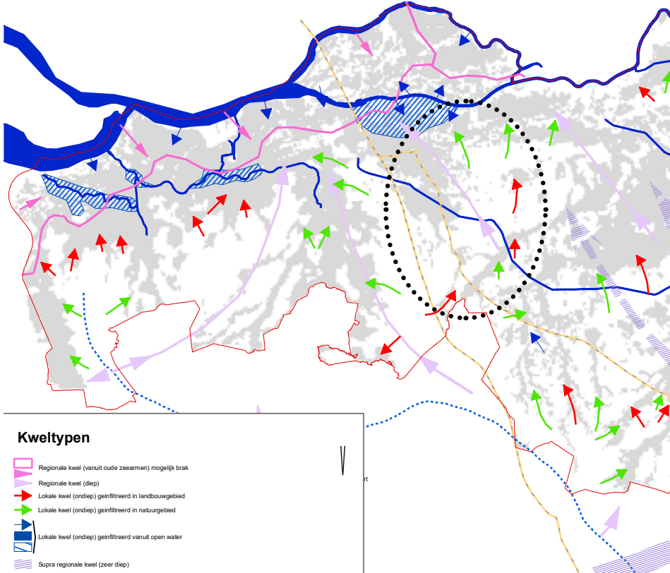
Kwel op regionale schaal
